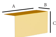
Bandeja 600 mm A: 600 mm B: 210 mm C: 287 mm
