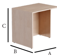
M8B 80 I A: 800 mm B: 600 mm C: 687 mm
