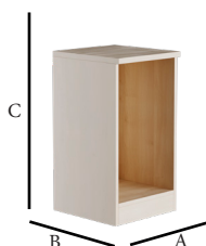
C 303 A: 400 mm B: 425 mm C: 745 mm
